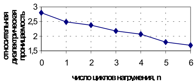
Рис. 3. а - Зависимость относительной диэлектрической проницаемости от числа циклов нагружения; алевролит, ш. 3. - Донбасская, гл. 480 м, "кубик"
