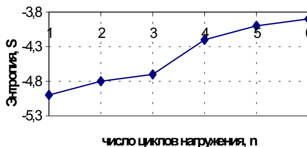
Рис. 3. в - Зависимость энтропии S от числа циклов нагружения; алевролит, ш. 3. - Донбасская, гл. 480 м, "кубик"
