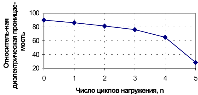
Рис. 1.а - Зависимость относительной диэлектрической проницаемости от числа циклов нагружения; уголь, ш. 3. - Донбасская, гл. 480 м, "балочка"
