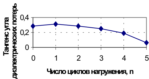
Рис. 1. б - Зависимость тангенса угла диэлектрических потерь от числа циклов нагружения; уголь, ш. 3.- Донбасская, гл. 480 м "балочка"
