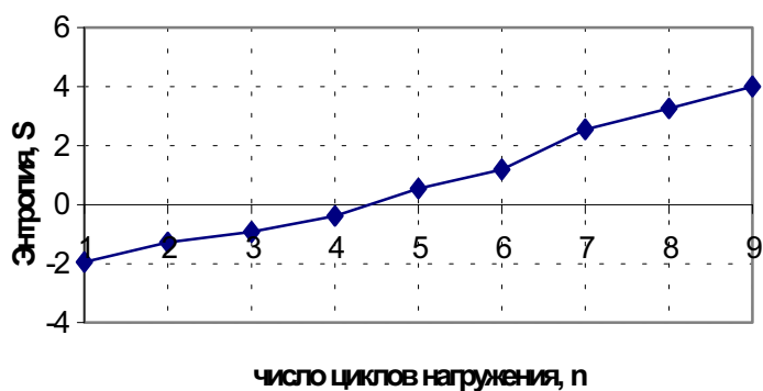
Рис. 2. в - Зависимость энтропии S от числа циклов нагружения; песчаник, ш. им. А. А. Скочинского, гл. 1100 м, "балочка"
