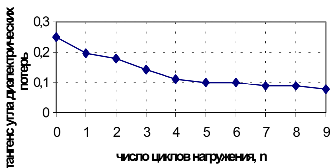
Рис. 2. б - Зависимость тангенса угла диэлектрических потерь от числа циклов нагружения; песчаник, ш. им. А. А. Скочинского, гл. 1100 м. "балочка"
